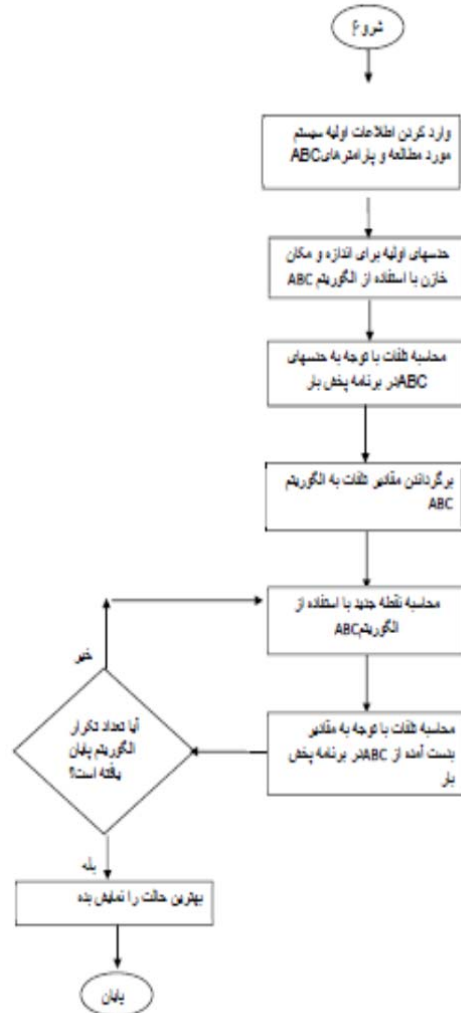
شکل ۳- فلوچارت الگوریتم زنبور عسل برای بهینه سازی اندازه و مکان خازن
