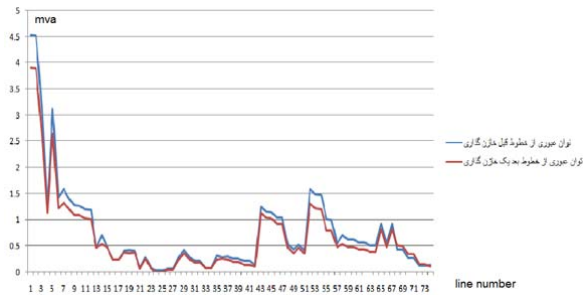
شکل ۷- توان عبوری از خطوط قبل و بعد از خازن گذاری
