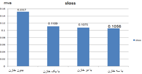
شکل ۵- نمودار تلفات در مراحل مختلف
