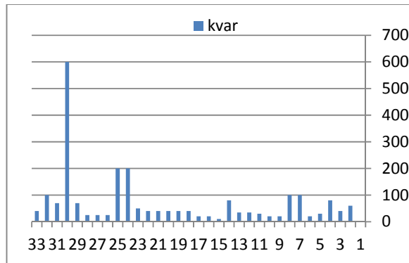
شکل ۴- نمودار توان راکتیو در شین های سیستم
