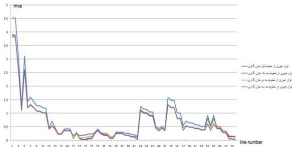
شکل ۸- توان عبوری از خطوط در حالت‌های مختلف خازن گذاری
