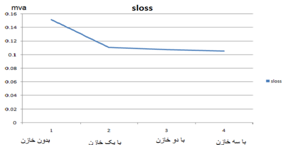
شکل ۶- اندازه تلفات در مراحل مختلف خازن گذاری
