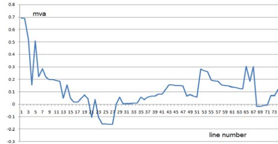
شکل ۹- ظرفیت آزاد شده خطوط در حالت بدون خازن و با سه خازن
