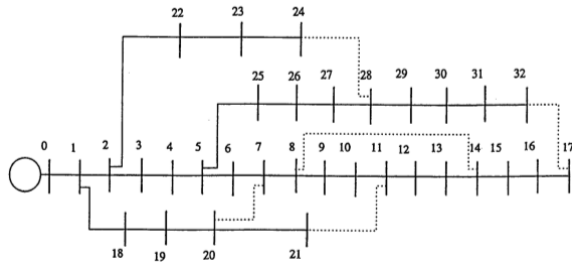
شکل ۱- شمای تک خطی سیستم ۳۲ باسه
